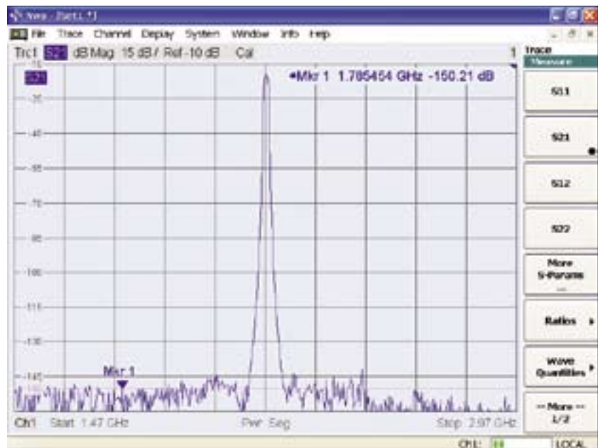
Номинальный динамический диапазон в режиме прямого доступа к приемнику
