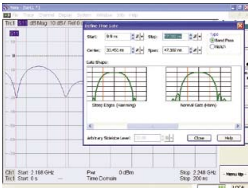
Настройка фильтра с помощью опции для измерений во временной области
