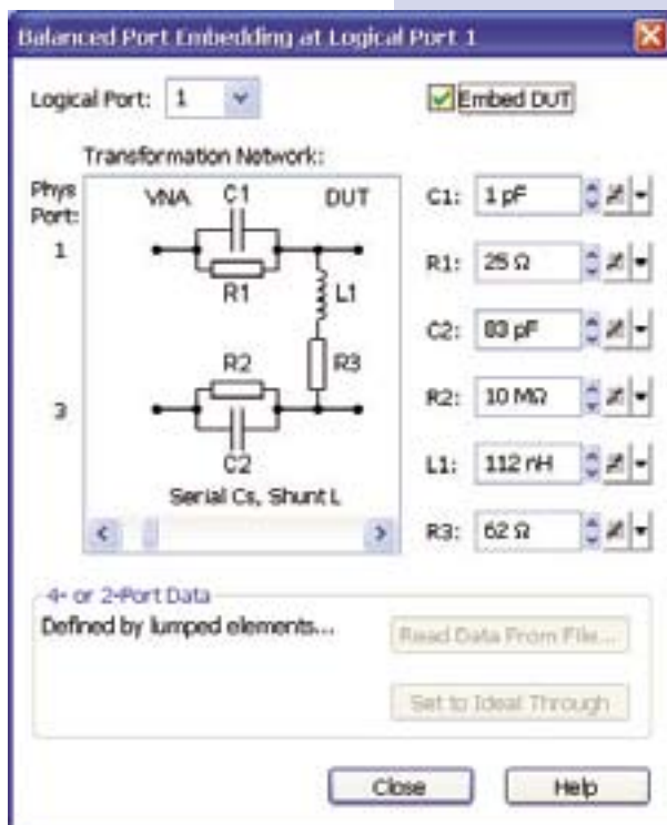
Параметризуемая цепь для виртуального согласования сопротивления
